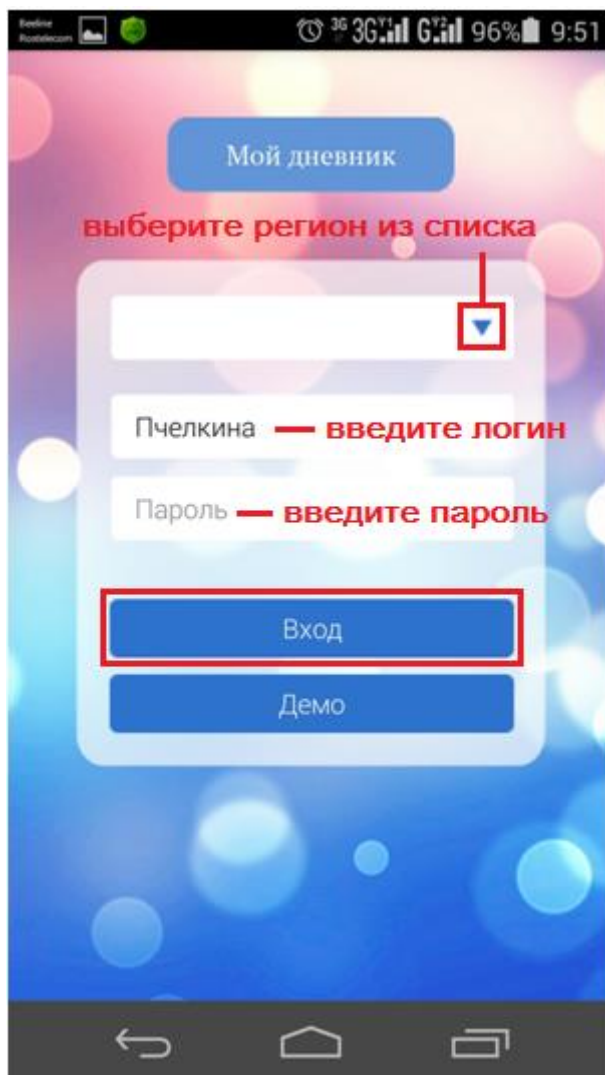
Рис. 1. Окно авторизации
